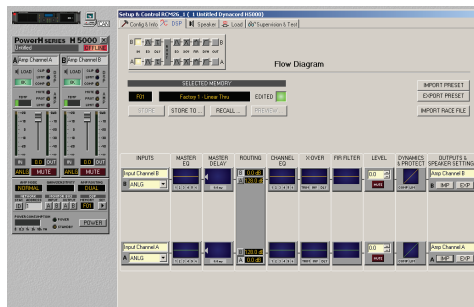
Illustration 4.2: Schéma de principe DSP du module RCM-26
